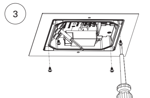
Deckenausschnitt / Ceiling cutout
